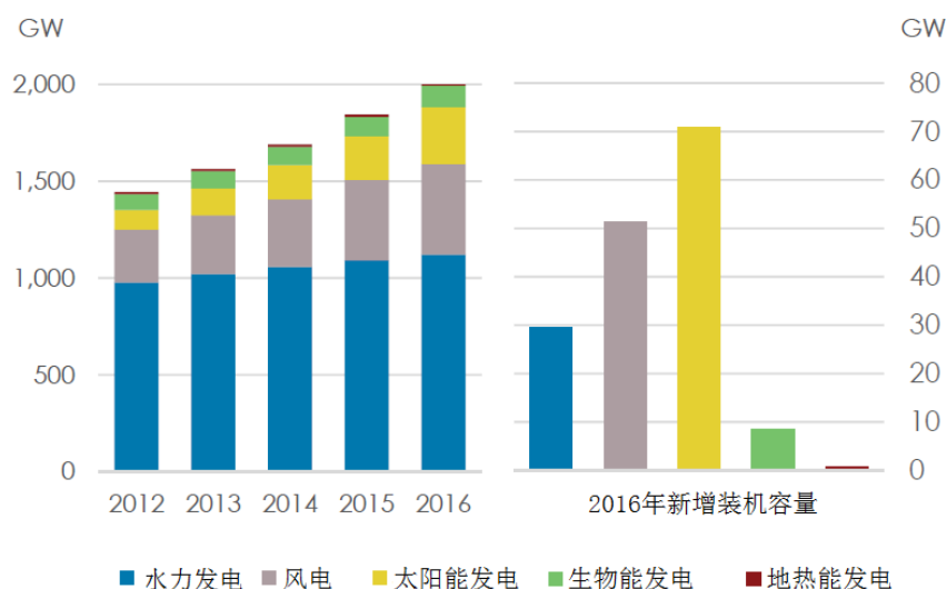
图 1 2012—2016 年可再生能源装机容量变化趋势
